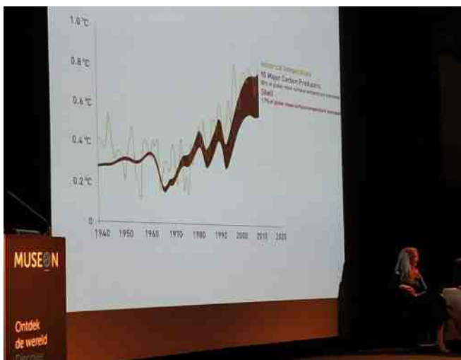
CO 2 -stijging en temperatuurstijging 1940-2020
